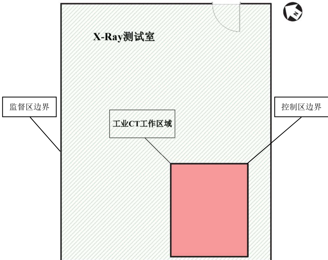
图 10-1 辐射工作场所平面布置图
