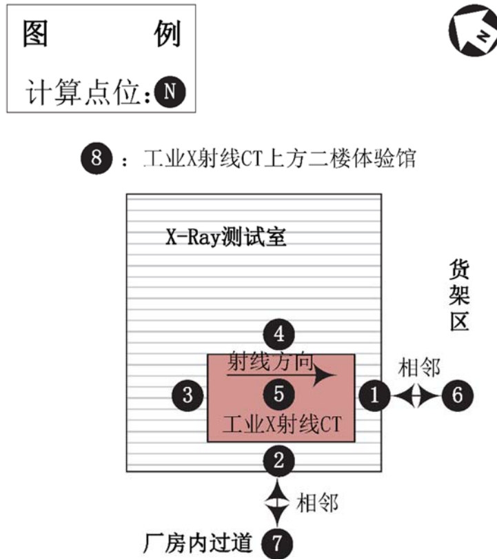
图 11-1 本项目工业 X 射线 CT 屏蔽计算点位示意图
