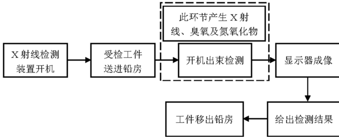
图 9-2 工业 X 射线 CT 工艺流程与产污环节示意图
