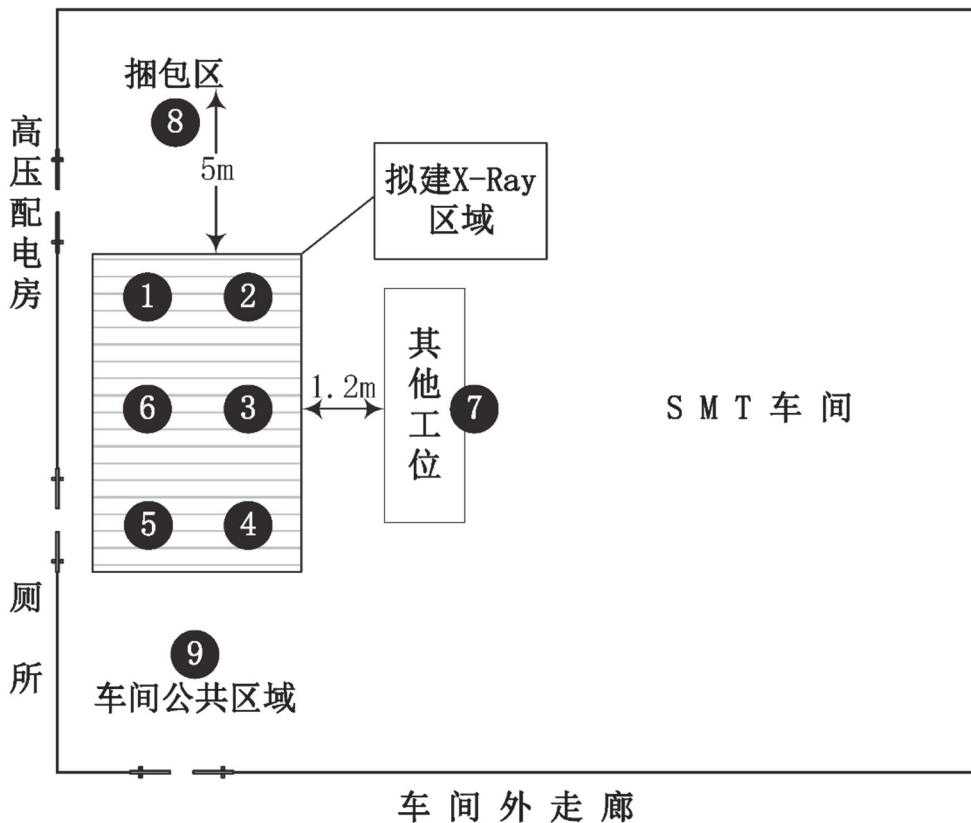
图 8-1 检测点位布置示意图
