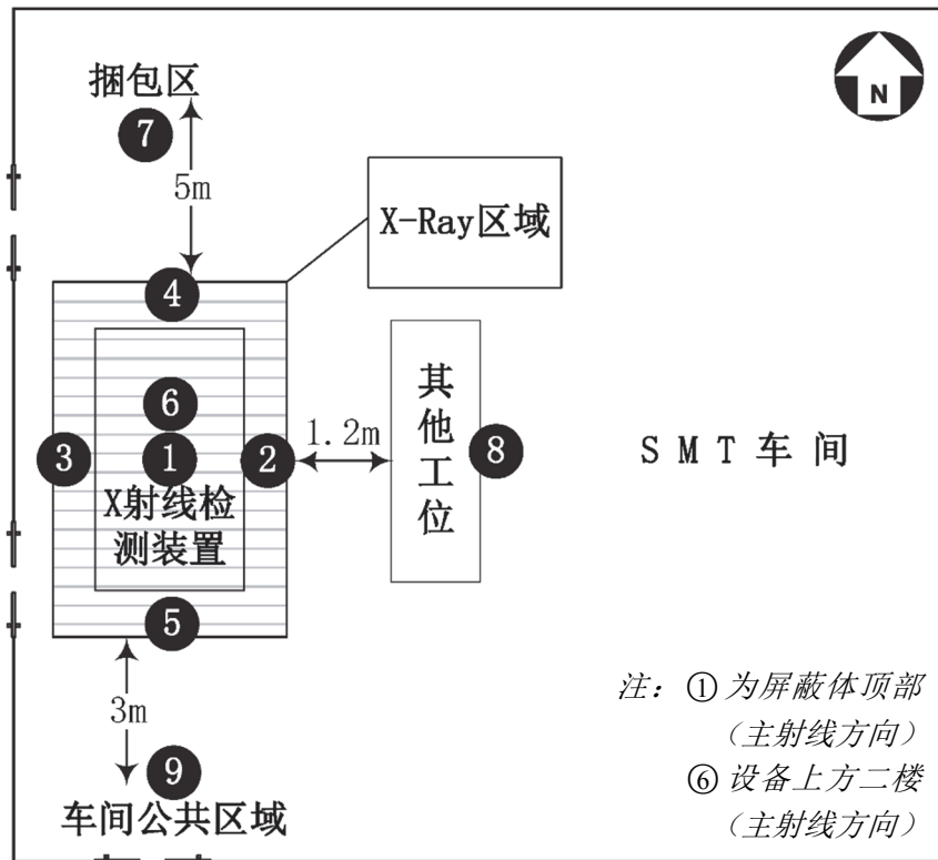
图 11-2 本项目 X 射线检测装置计算点位分布示意图
